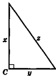
Пифагоров треугольник
