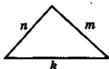
Целочисленный треугольник
