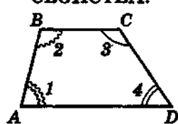
ABCD – трапеция
