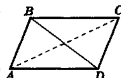
ABCD — параллелограмм
