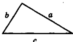
Разностный треугольник
