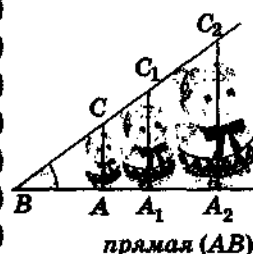
прямая ( AB )
