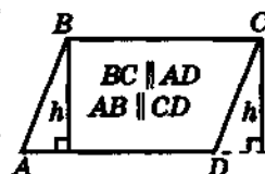
h — высота
