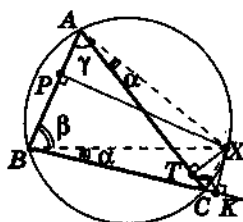
Теорема Симпсона
