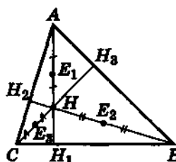
Точки Эйлера
